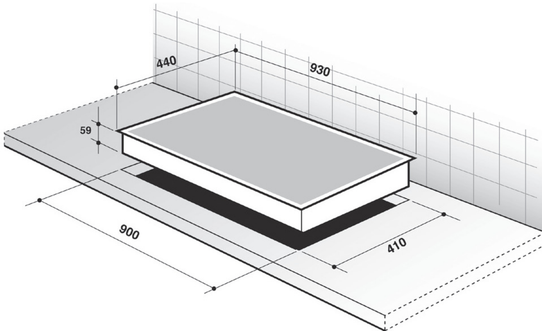
安裝圖
